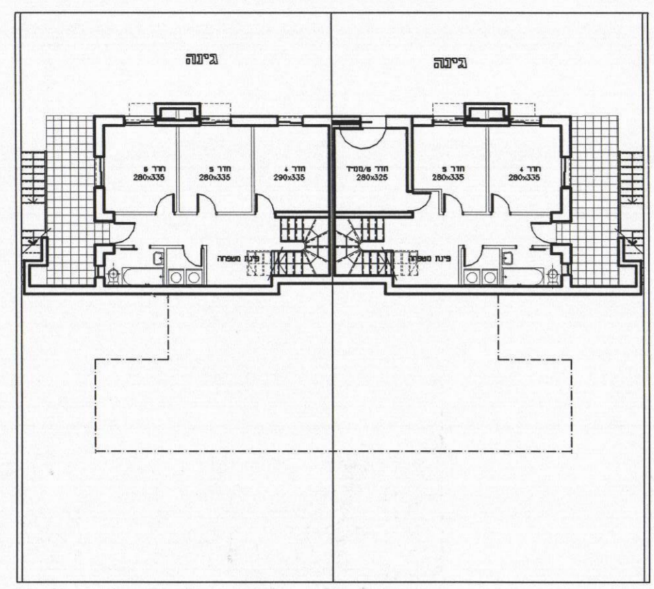
קומה 2 - מפלס 00.5 גר' / קומה 2 - מפלס 00.5 גר'
