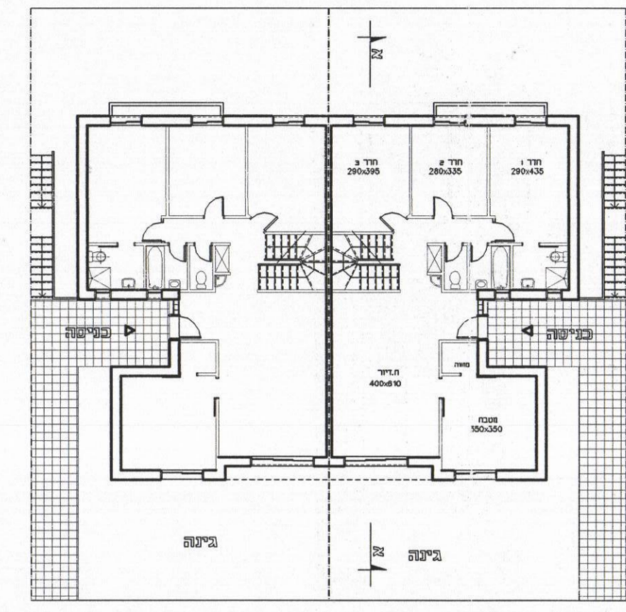
קומה 6 - מפלס 03.00 גר' / קומה 6 - מפלס 03.00 גר'
