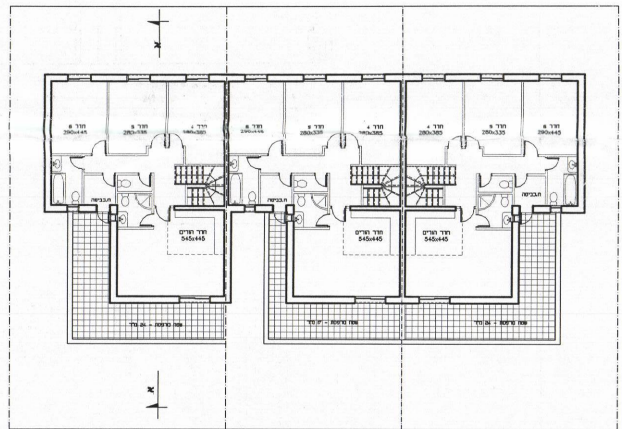
קומה - מפלס עליון 00 גר' / תוכנית - מפלס עליון 00 גר' / תוכנית - מפלס עליון 00 גר'
