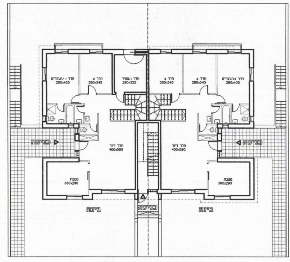
קומה 3 - מפלס 00.00 גר' / קומה 3 - מפלס 00.00 גר'
