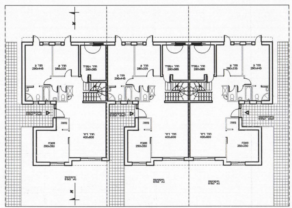
קומה - מפלס כניסה 000 גר' / תוכנית - מפלס כניסה 000 גר' / תוכנית - מפלס כניסה 000 גר'
