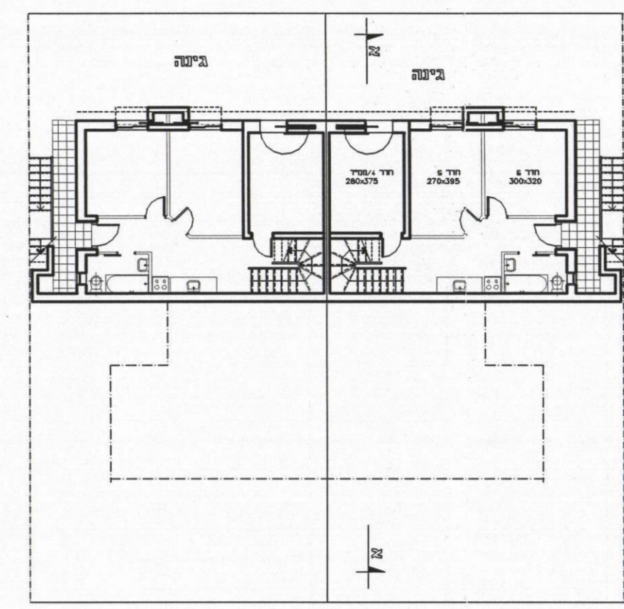
קומה 5 - מפלס 02.50 גר' / קומה 5 - מפלס 02.50 גר'
